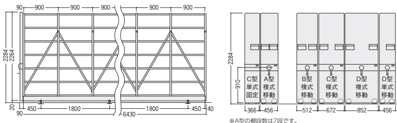
●7連式正面図
